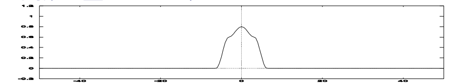
スペクトルに矩形関数を乗じたもの=原スペクトルと同じスペクトル これは標本値パルス列とsinc関数の畳み込みに相当
